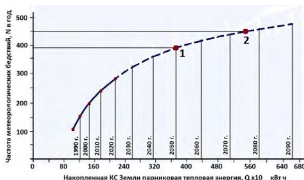
Рис. 8. График зависимости частоты повторяемости метеорологических стихийных бедствий (М-бедствий) от накопленной тепловой энергии в КС Земли: 1 – частота М-бедствий в 2050 г.; 2 – максимальная частота N = 450 ед/год
